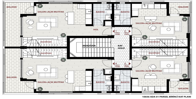
10656 ADA 01 PARSEL BİRİNCİ KAT PLANI
